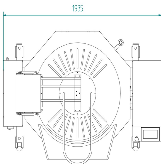
VISTA PLANTA
